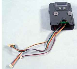
Control Module KW710750 Timer PCB KW714103
